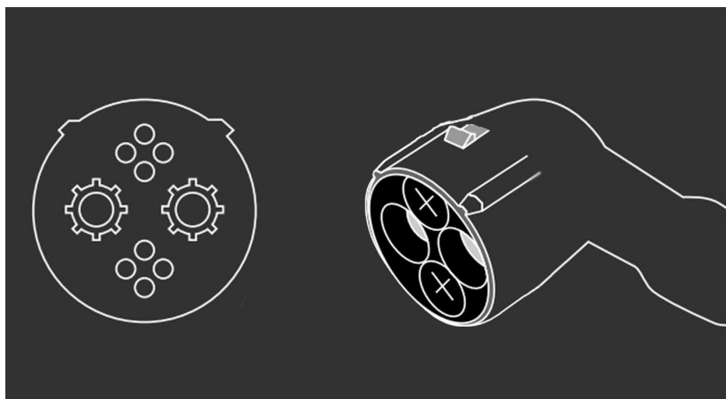
Pistola CHAdeMO
